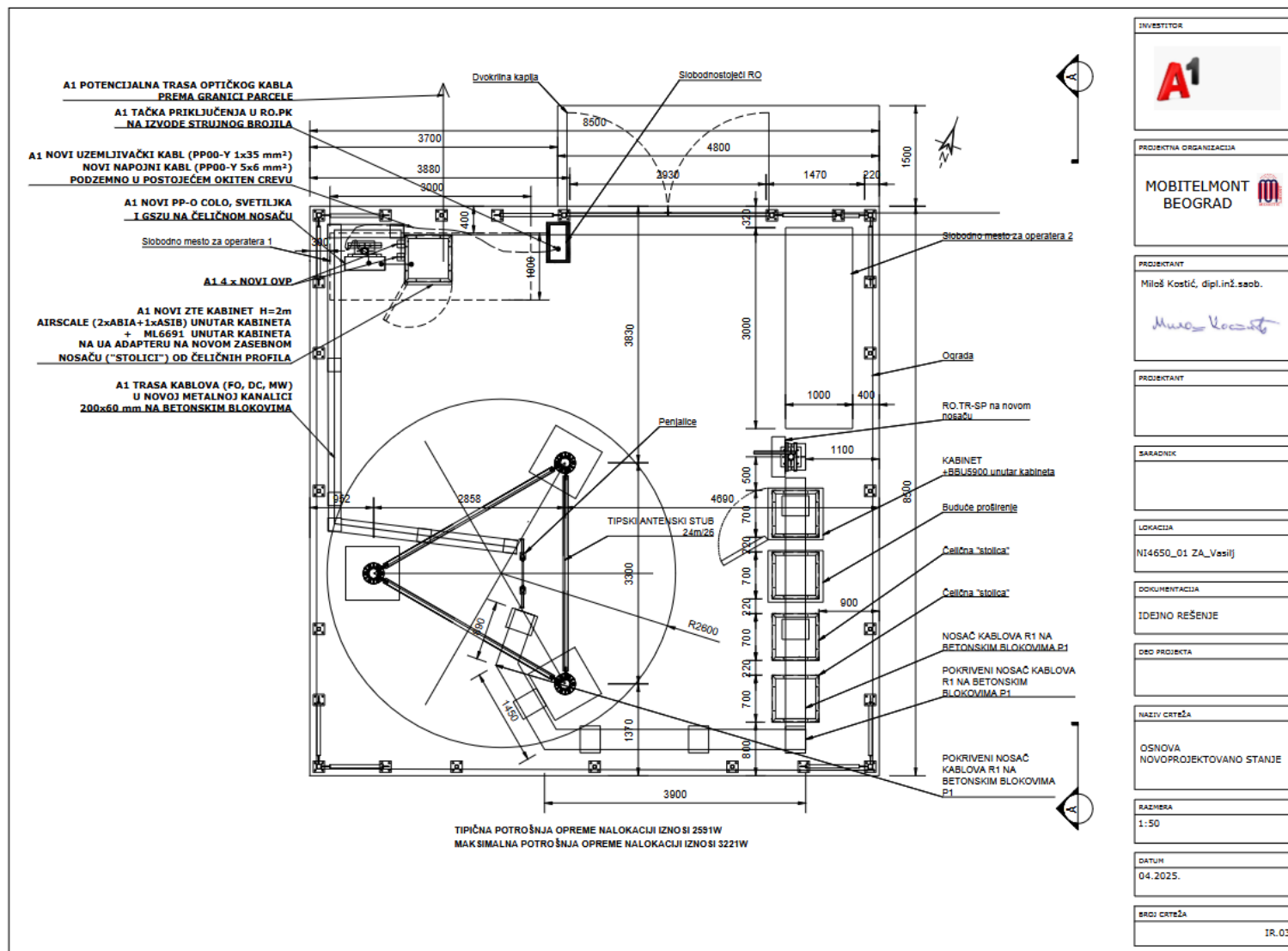
Слика 8.1. Ново стање на локацији – Основа
