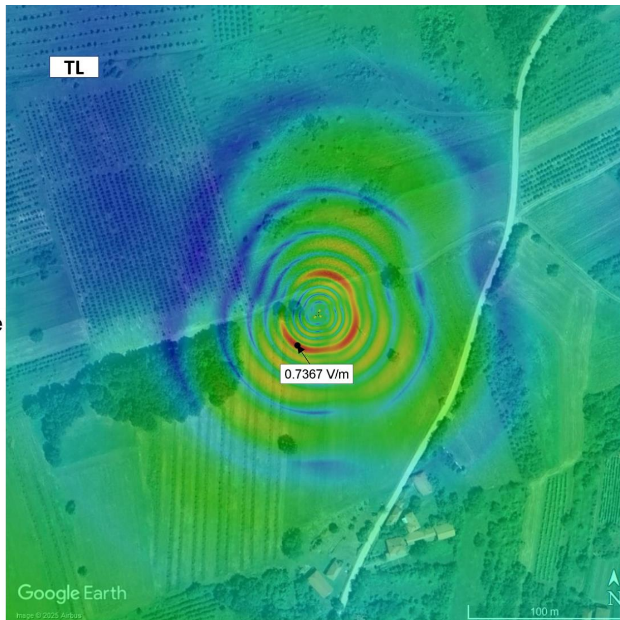
Слика 4.5. Јачина електричног поља на јавном подручју (на тлу), када радио-систем LTE2100 оператора А1 Србија ради максималним капацитетом
