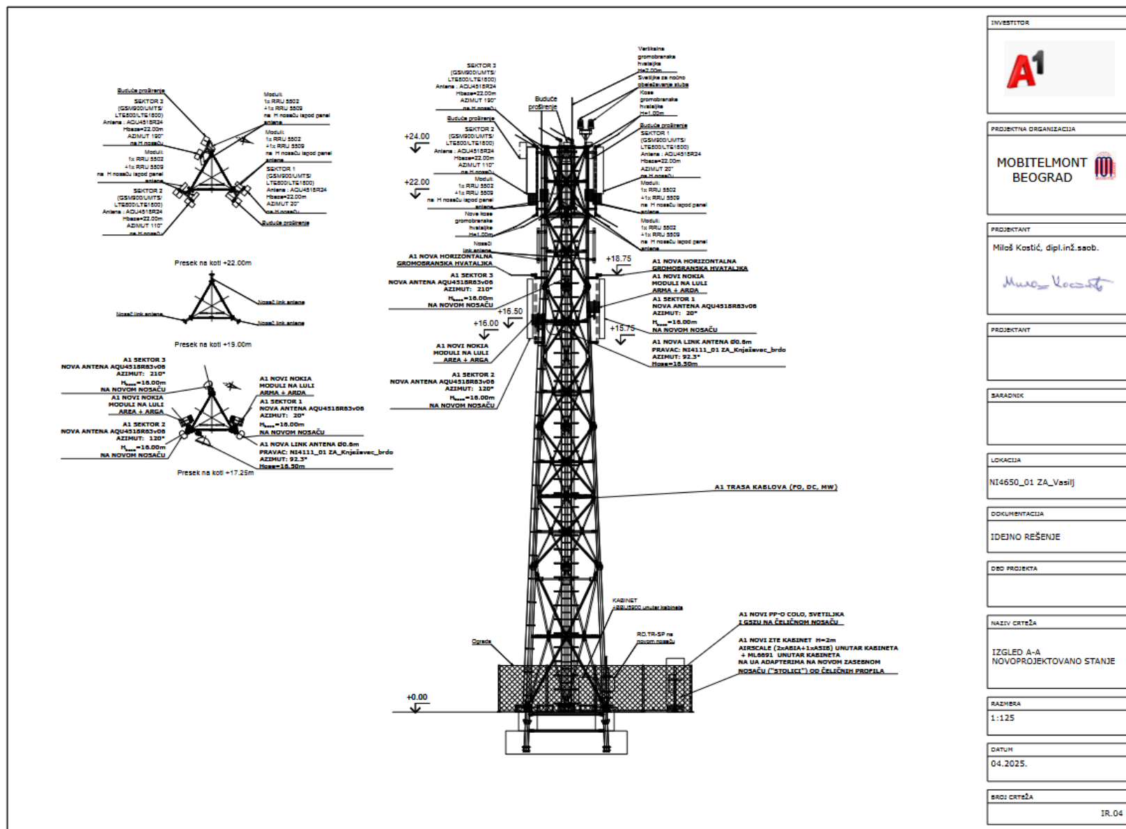
Слика 8.2. Ново стање на локацији – Изглед А-А
