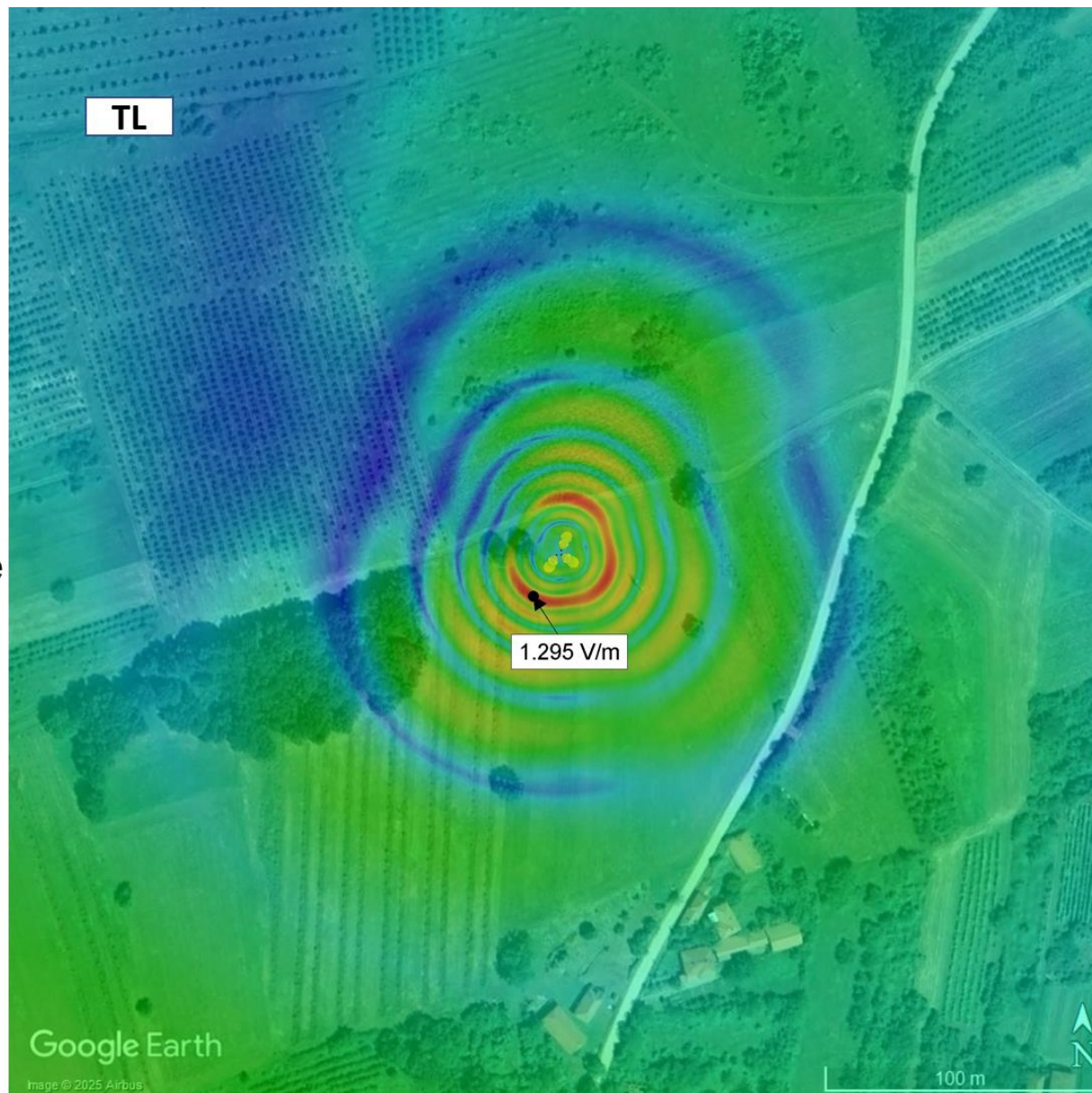
Слика 4.4. Јачина електричног поља на јавном подручју (на тлу), када радио-систем LTE1800 оператора А1 Србија ради максималним капацитетом
