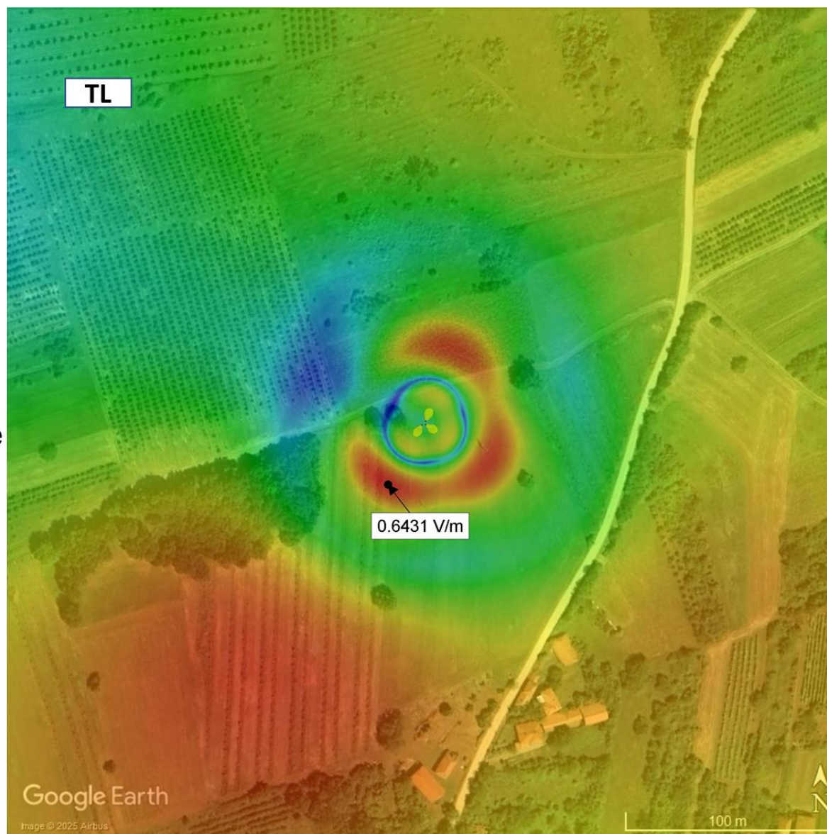
Слика 4.2. Јачина електричног поља на јавном подручју (на тлу), када радио-систем GSM900 оператора А1 Србија ради максималним капацитетом
